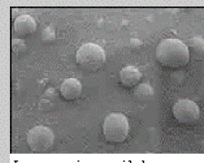
Las rocas sin rugosidades son una de las pruebas de que hubo agua en Marte
